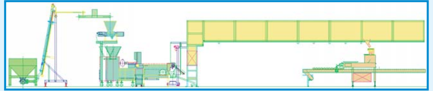
ドゥポンプ DO PUMP ドゥフロー DO FLOW 分配器 DISTRIBUTOR 分割丸め機 DIVIDER ROUNDER プルーファ PROOFER モルダパンナ MOULDER PANNER
